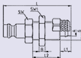
Bulkhead Fitting for Kunststoffschlauch
